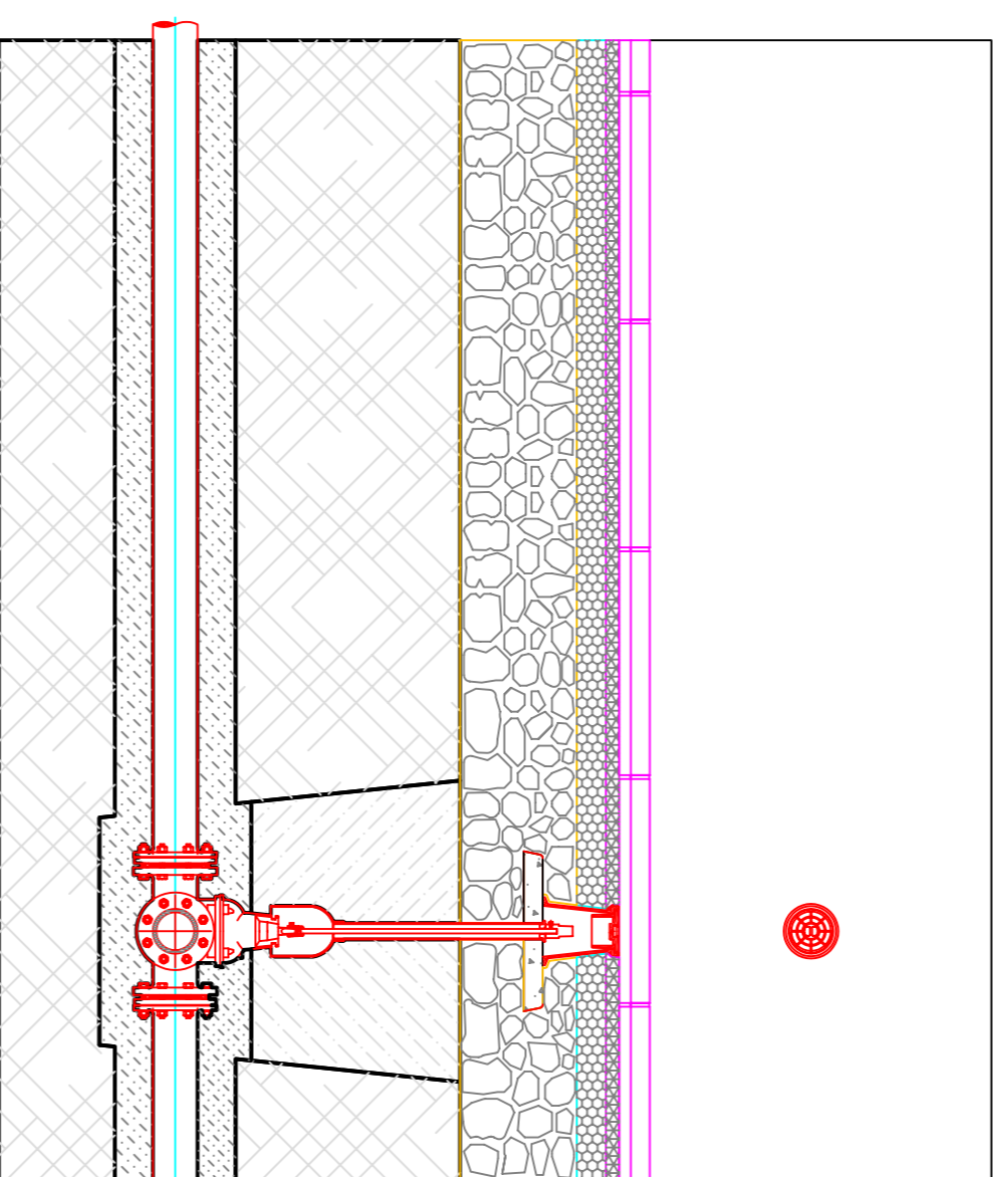
Derivazione da condotta adduttice con saracinesca d'intercettazione sottosuolo
