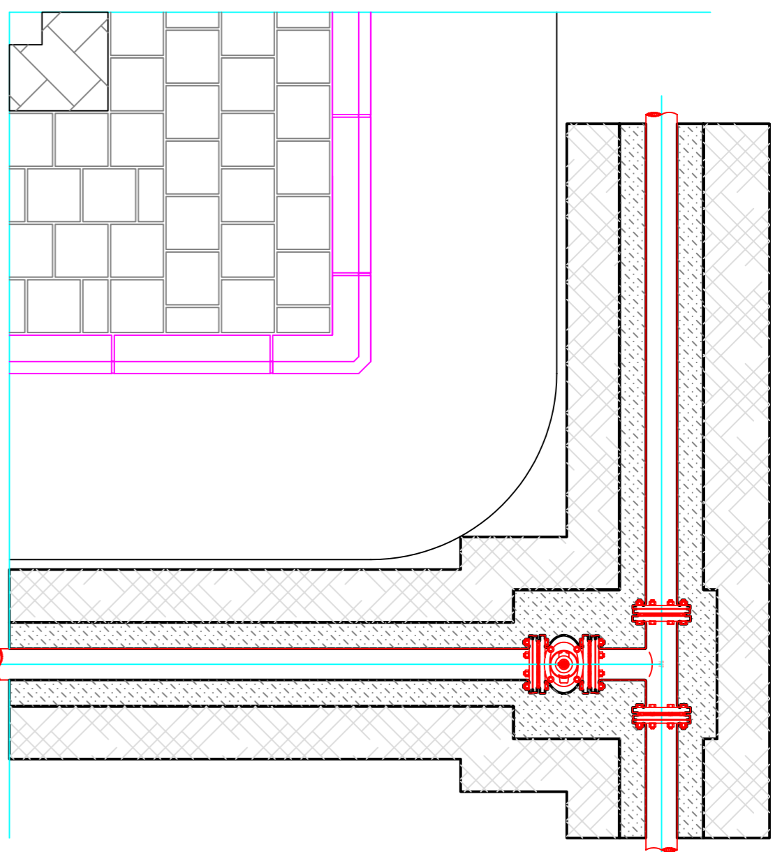
Derivazione da condotta adduttice con saracinesca d'intercettazione sottosuolo
