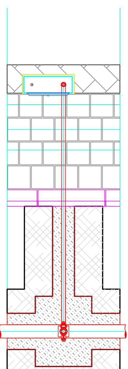
Derivazioni allacci privati con collare di presa
